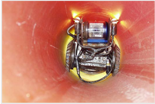
Abbildung 32 | Robotersanierung
