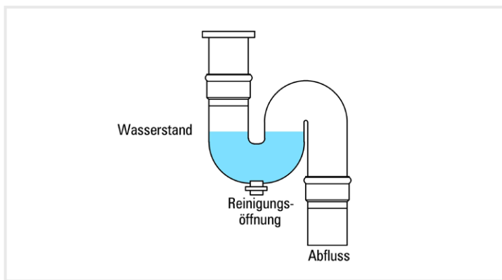
Abbildung 3 | Geruchsverschluss
