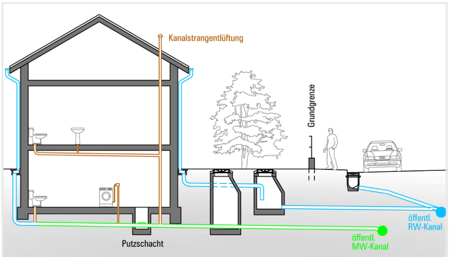
Abbildung 11 | Qualifiziertes Mischsystem
