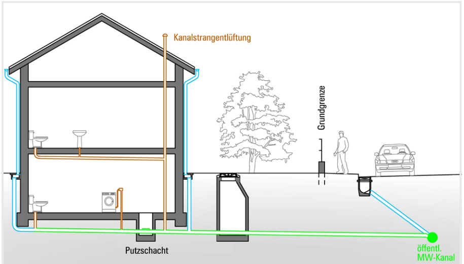
Abbildung 10 | Mischsystem
