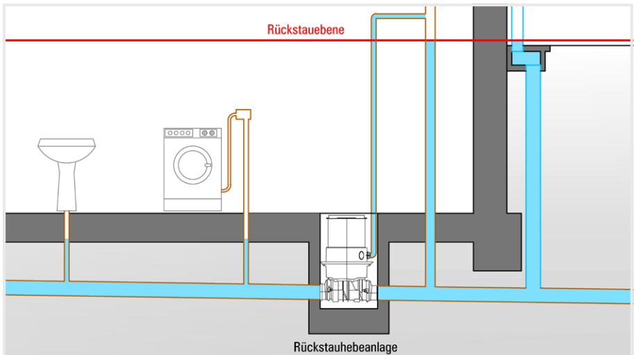
Abbildung 7 | Rückstauhebeanlage
