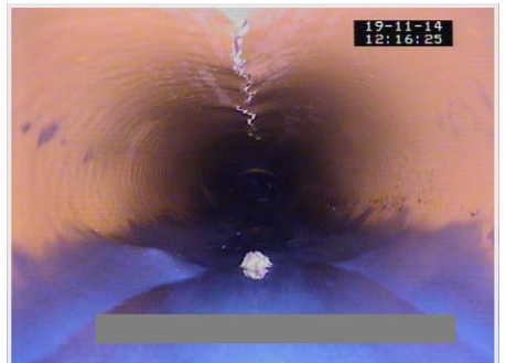
Abbildung 25 | Rohrbruch
