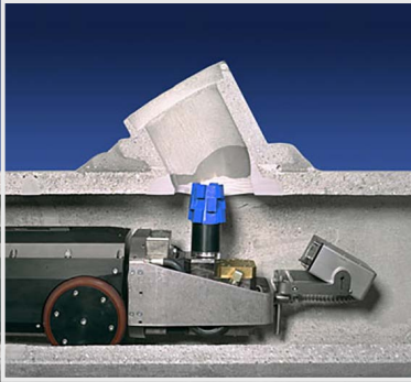
Abbildung 31 | Robotersanierung
