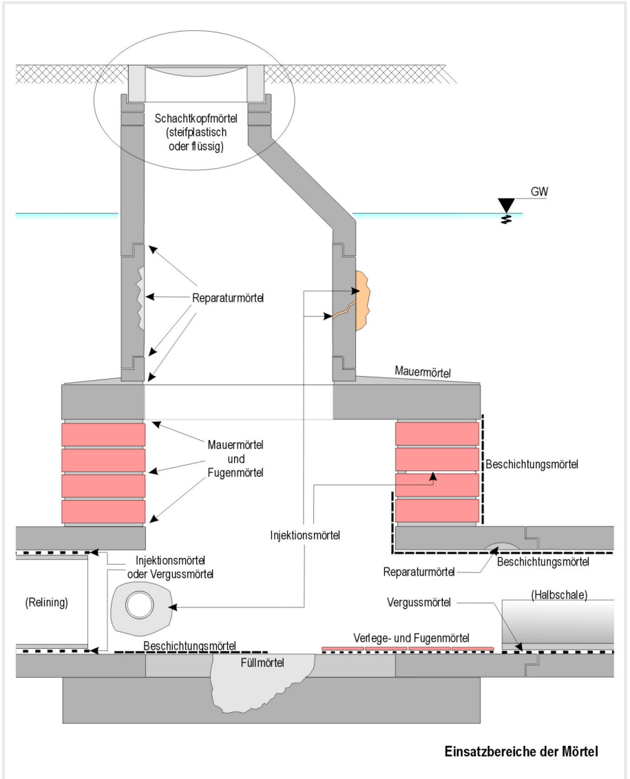
Abbildung 35 | Schachtsanierung
