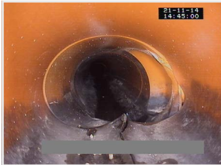
Abbildung 26 | Rohrbruch Kanalsohle
