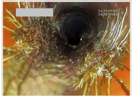
Abbildung 23 | Durchwurzelung
